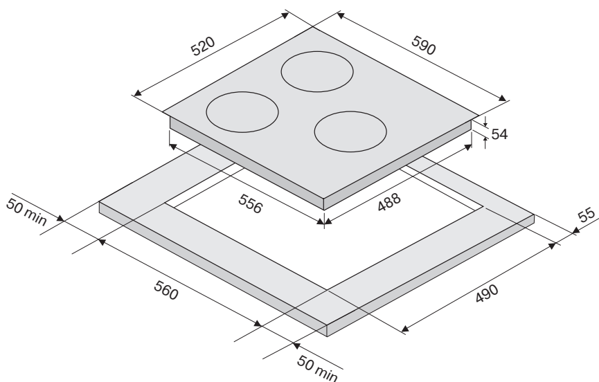
Схема встраивания варочной поверхности
